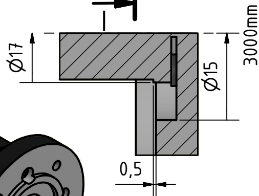
SNITT I-I
